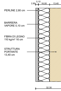
SCALA 1:10 PARETE BLOCKHOUSE ESTERNA ASIAGO
