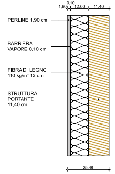
SCALA 1:10 PARETE BLOCKHOUSE ESTERNA BASSANO
